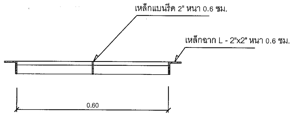
รูปตัดฝากรอบรางระบายน้ำ
