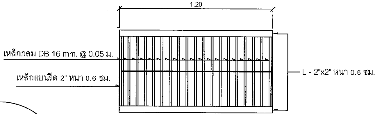
แบบแปลนฝากรอบรางระบายน้ำ
