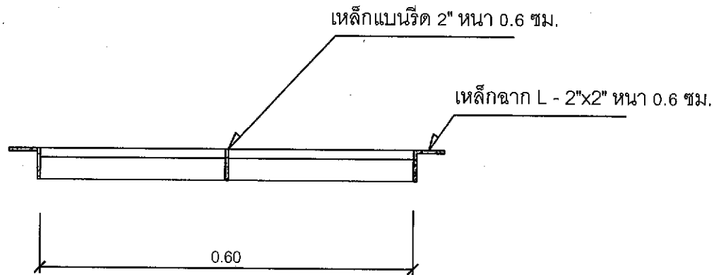
รูปตัดฝักรอบรางระบายน้ำ
