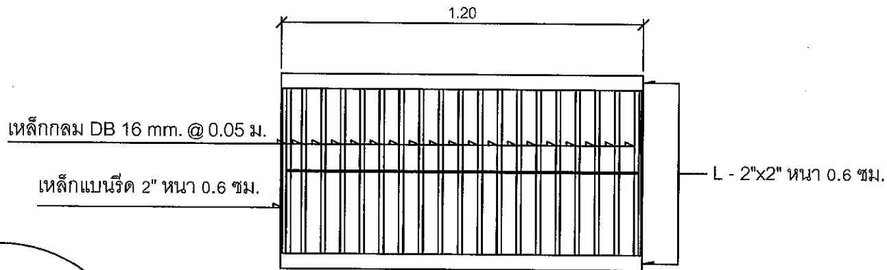
แบบแปลนฝักรอบรางระบายน้ำ
