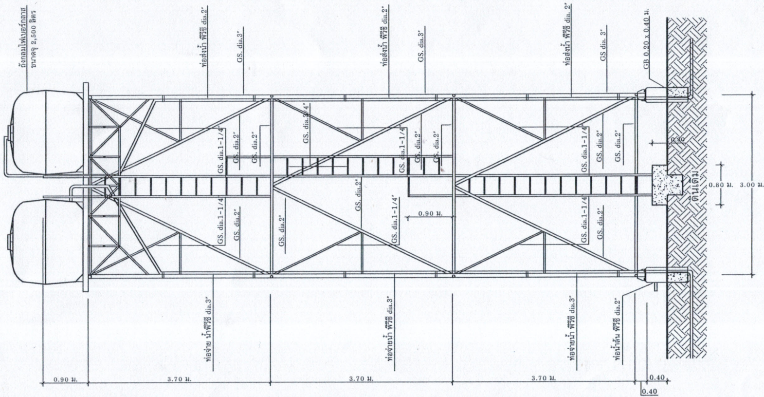
รูปตัดขยายท่อส่งโครงเหล็ก
