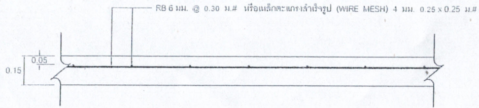
แบบขยายการเสริมเหล็กตะแกรง
