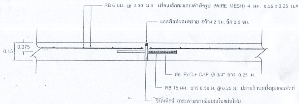
แบบขยายรอยต่อเพื่อการขยายตัว (EXPANSION JOINT)
