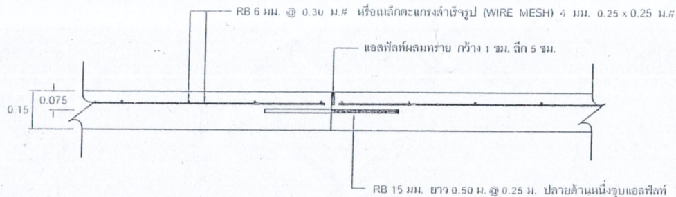
แบบขยายรอยต่อเพื่อการหดตัว (CONTRACTION JOINT)
