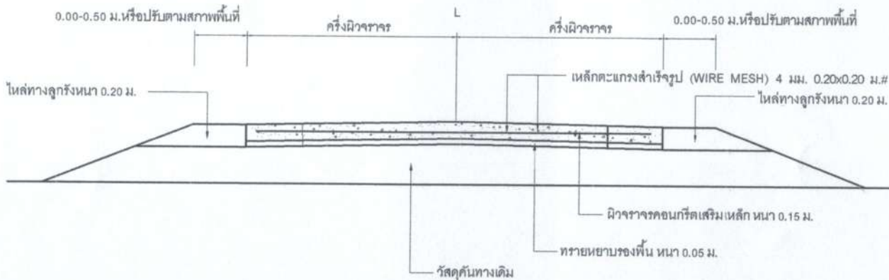
รูปตัด ก-ก Not To Scale
