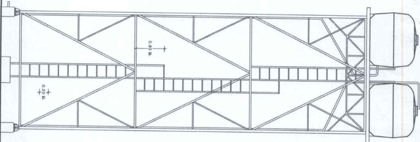
รูปด้าน มาตราส่วน 1 : 1 : 50
