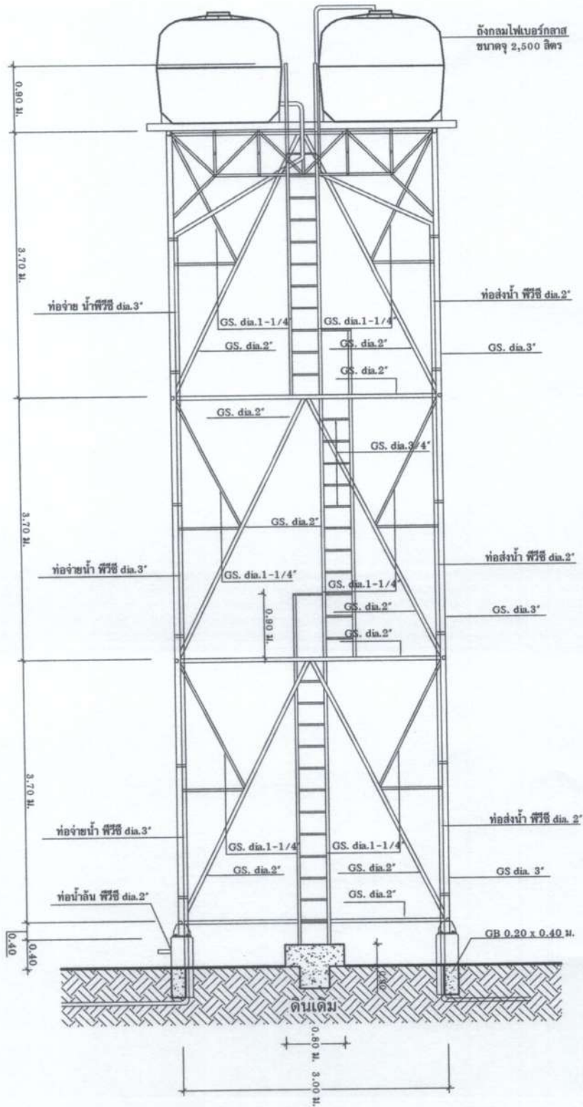
รูปตัดขยายหอดังโครงเหล็ก
