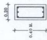
ขยายคาน GB ขนาดชั้น 1 : 80
