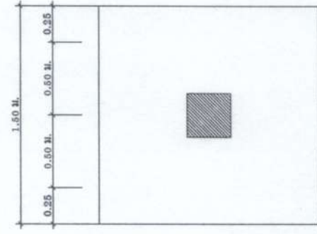
แปลนขยายฐานราก ขนาดชั้น 1 : 25
