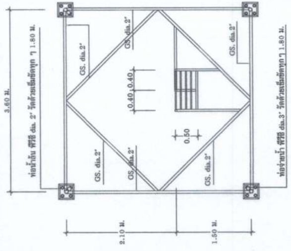
แปลนชั้นที่ 2 ขนาดส่วน 1:50
