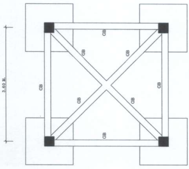
แปลนฐานราก คานคอดิน ขนาดชั้น 1 : 80
