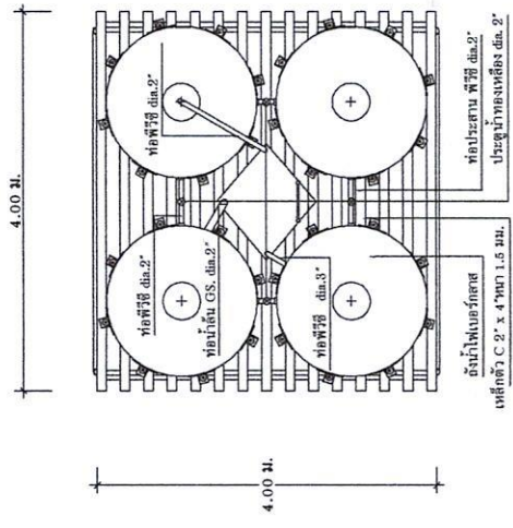
แปลนชั้นรับถังน้ำ ขนาดส่วน 1 : 100
