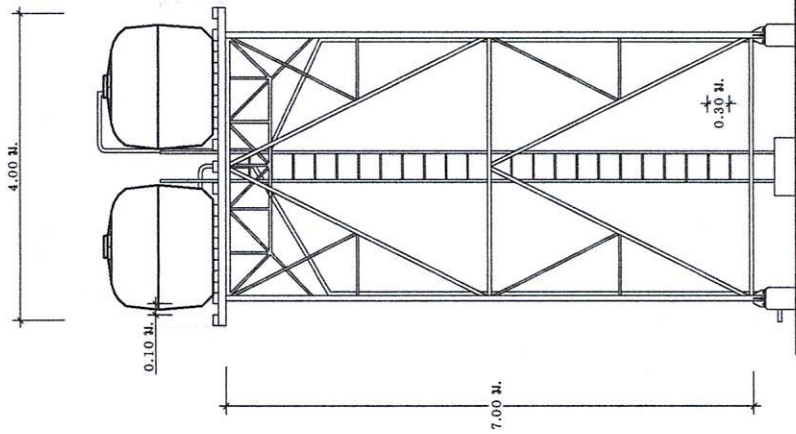
รูปด้าน ขนาดส่วน 1 : 100
